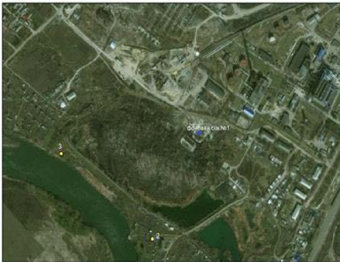
Ситуационный план размещения наблюдательных скважин на территории зона отвода ПП "Ливенская ТЭЦ" филиала ПАО "Квадра"- "Орловская генерация"
